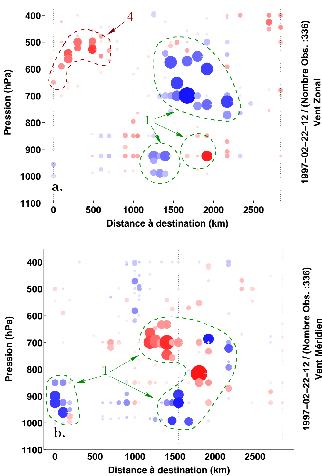
FIG. 5.13: Contributions à l'impact sur la fonction coût \mathcal{J} (enstrophie) par les observations ciblées de vent. (a.) représente les éléments de \mathcal{J}_{C_t} (cf. équation 5.4) correspondant à la composante zonale du vent; (b.) contient les éléments relatifs à la composante méridienne. Les valeurs extrêmes des contributions par le vent zonal sont: Max \simeq 8.5 \times 10^{-8} s^{-2} et min \simeq -1.2 \times 10^{-7} s^{-2} . Les valeurs extrêmes des contributions dues au vent méridien sont: Max \simeq 1.2 \times 10^{-7} s^{-2} et min \simeq -9.0 \times 10^{-8} s^{-2} . Les structures remarquables entourées de tirets numérotées 1 correspondent à des zones de sensibilité marquée sur la figure (5.11). La zone notée 4 relève d'une sensibilité plus modérée.
