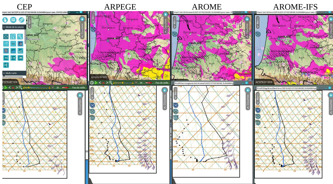
Run 27/02/2020 00UTC pour le samedi 29 00UTC
