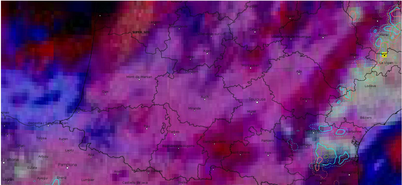
Eau nuageuse à 10m (Aromes) ou 20m (Arpège) valide le 13/01 à 08UTC avec (ARPEGE /AROME-fr/AROME-IFS) de J 00H.
